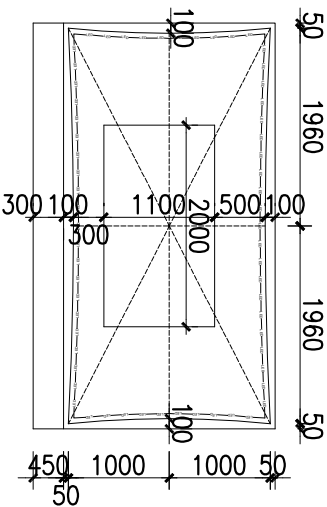
电视背景墙平面
