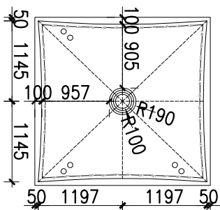
餐厅天花造型
