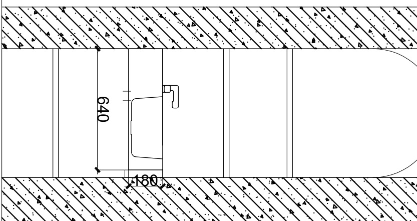
主卫洗手台(台面出水)定制立面图
